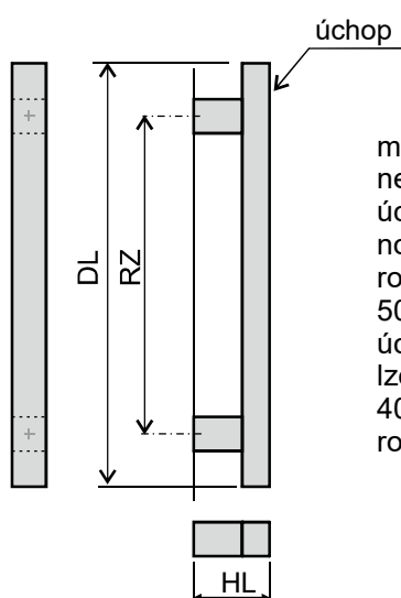
zobrazený model typ FHR30x20-500/350 bez podložek
