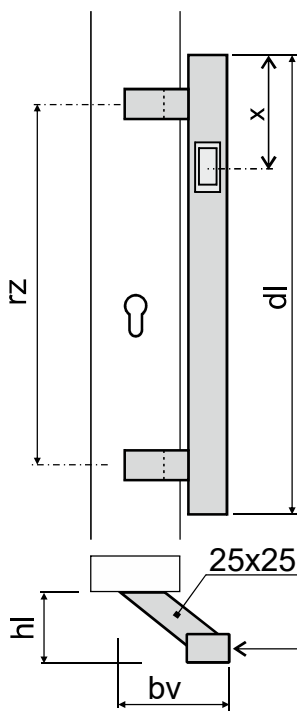
Rozměry rz, dl, x jsou volitelné
