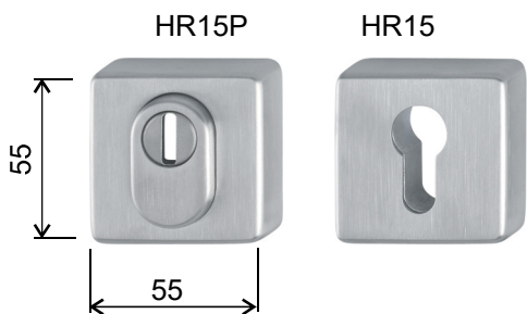
venkovní krycí zámkové rozety hranaté pro doplnění kliky a madla
